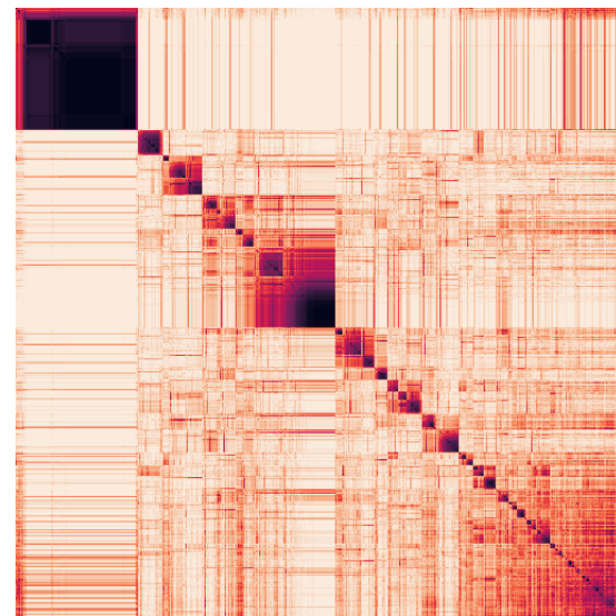
tp17 (PAC=0.33, 2000 genes)
